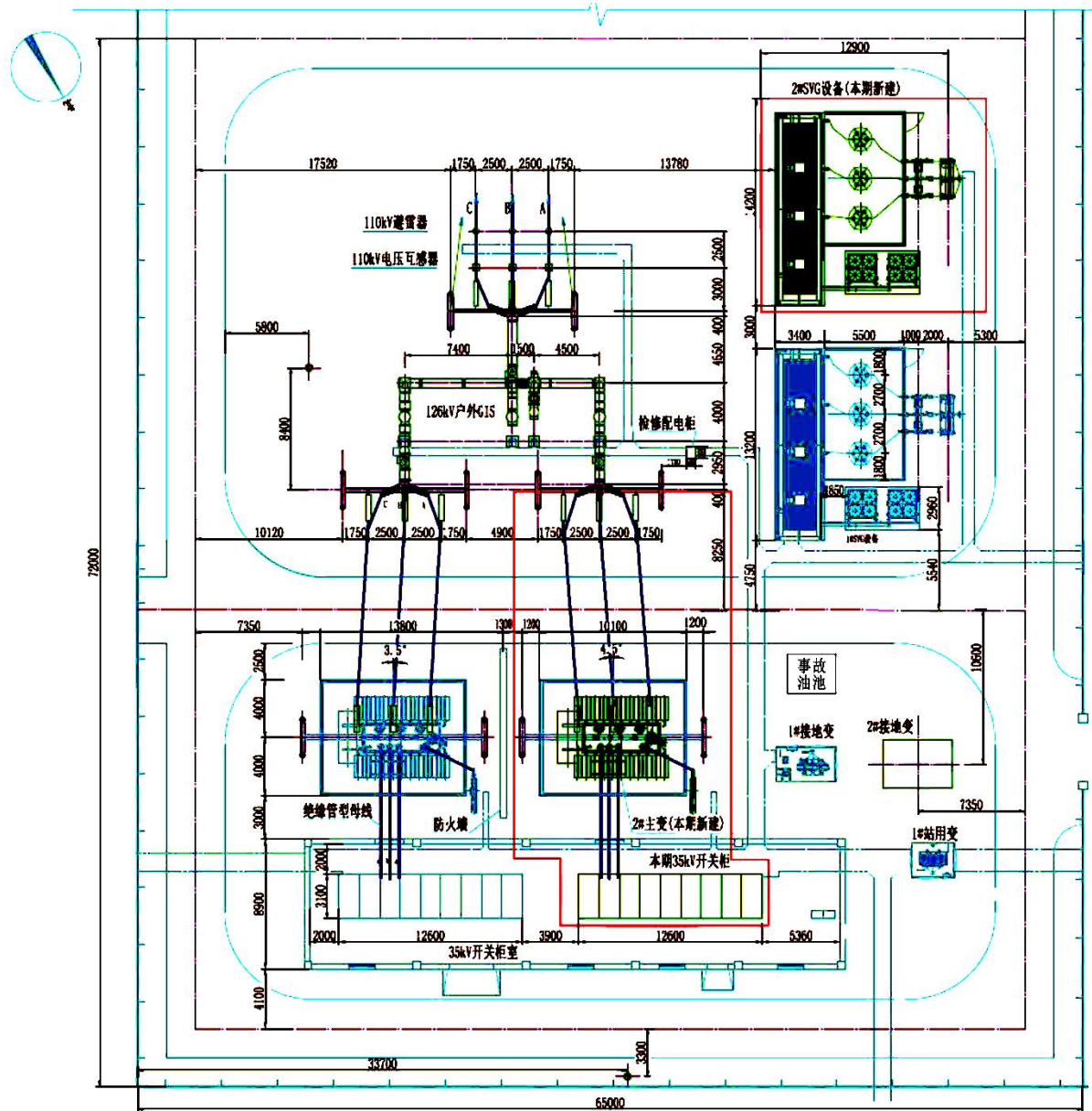
图 1 贺圈新墩风电场 110kV 升压站工程平面布置图
